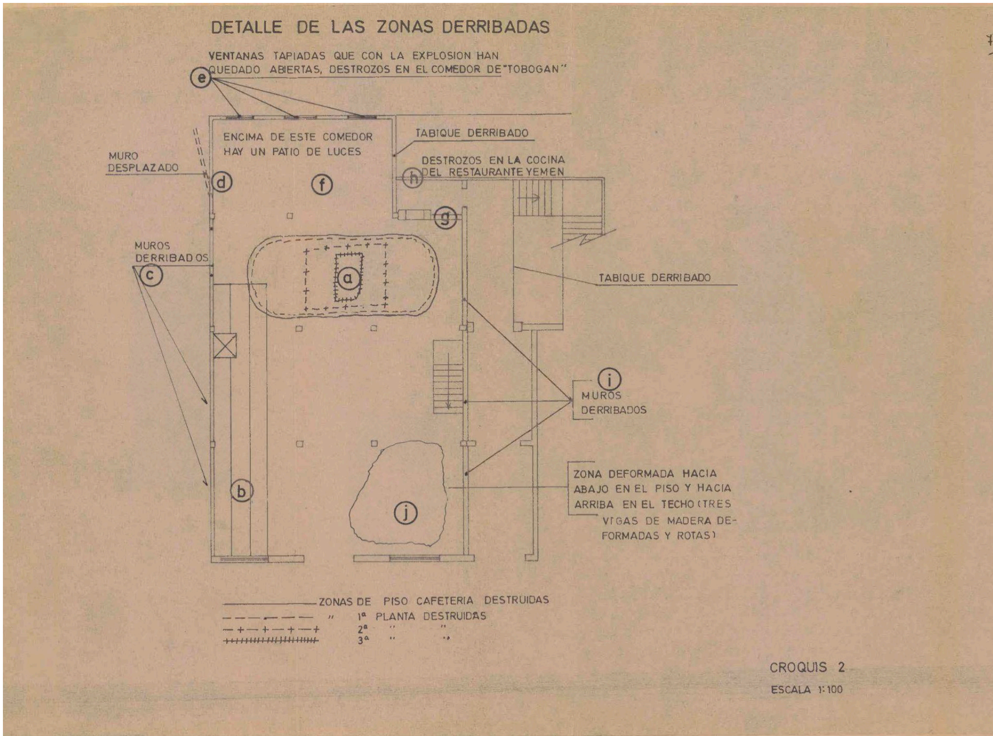
Plano de la cafetería Rolando tras la explosión elaborado por el Parque y Maestranza de Artillería de Madrid. Fuente: Archivo Judicial Territorial de la Comunidad de Madrid, Sumario 2/1977 del Juzgado de Instrucción nº 21 de Madrid.
